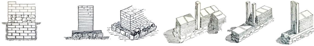
Şekil.1: Geleneksel konutlardaki duvar yapım teknikleri (Nauman, 1975,62-110)
